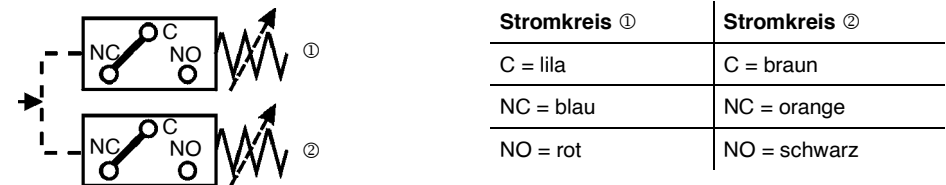
Bild 5: Schalt- und Anschlusschema
