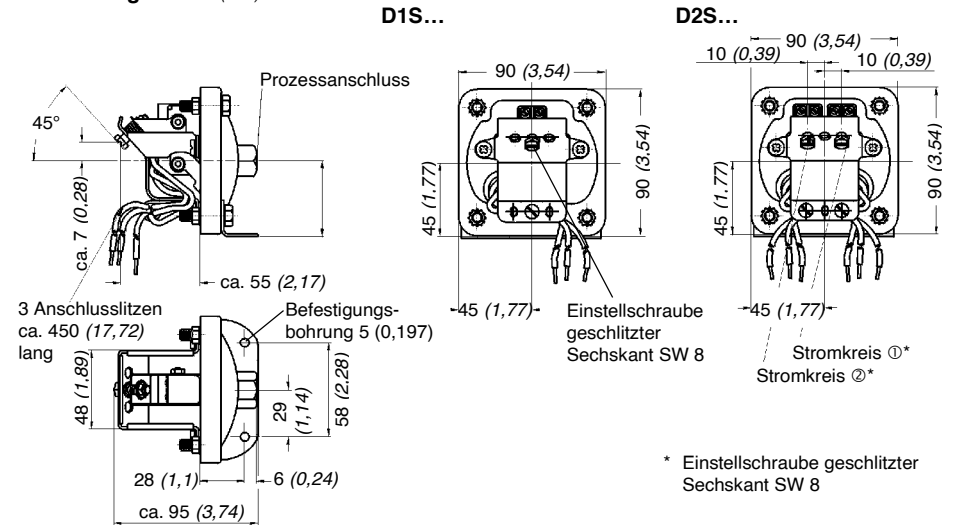
Bild 7: Metall-Membran-Druckschalter Typ D1S .../D2S ...
