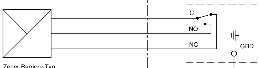
Zener-Barrier-Typ Schaltverstärker NAMUR
