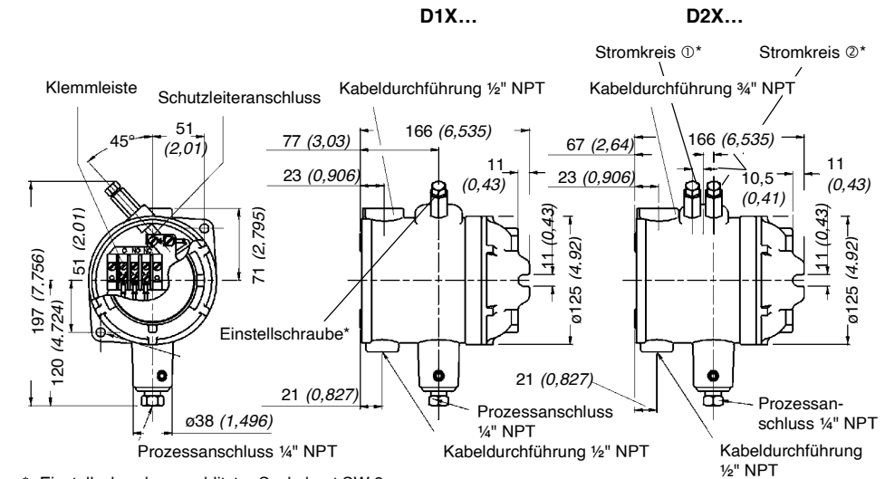
Bild 8: Metall-Membran-Differenz-Druckschalter Typ D1X .../D2X ...
